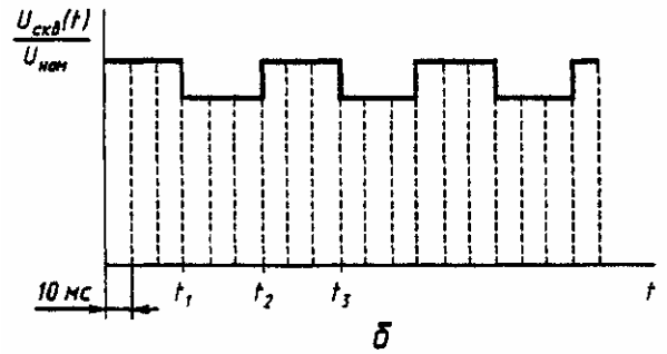
Рисунок Б.1 — Колебания напряжения произвольной формы (а) и имеющие форму меандра (б)
