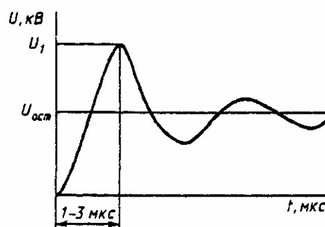
Рисунок Д.2 — Форма грозовых импульсов, характерная для точек присоединения а, е, г, д на рисунке Д.1.
