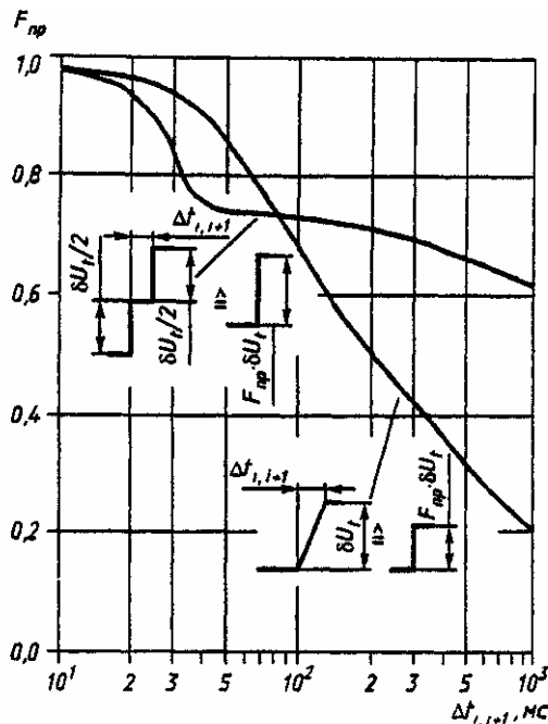
Рисунок В.1 — Коэффициент приведения F_{\text{пр}} для периодических колебаний напряжения, имеющих двухступенчатую и пилообразную форму
