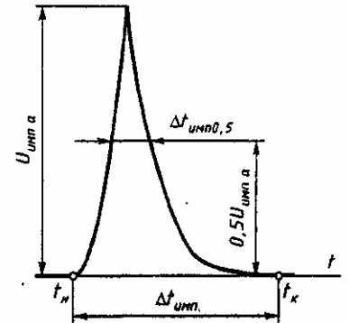
Рисунок Б.3 — Параметры импульсного напряжения
