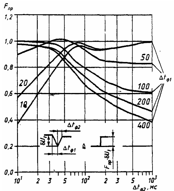
Рисунок В.3 — Коэффициент приведения F_{\text{пр}} для периодических колебаний напряжения, вызванных пуском двигателей
