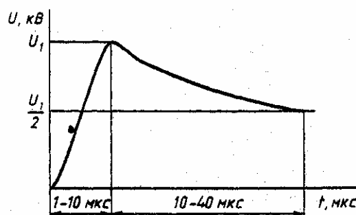
Рисунок Д.4 — Форма грозовых импульсов, характерная для точек присоединения б, в, ж на рисунке Д.1.
